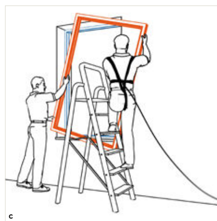
c Le nouveau dormant est ensuite simplement appliqué par dessus l'ancien cadre, sur lequel il est vissé.
